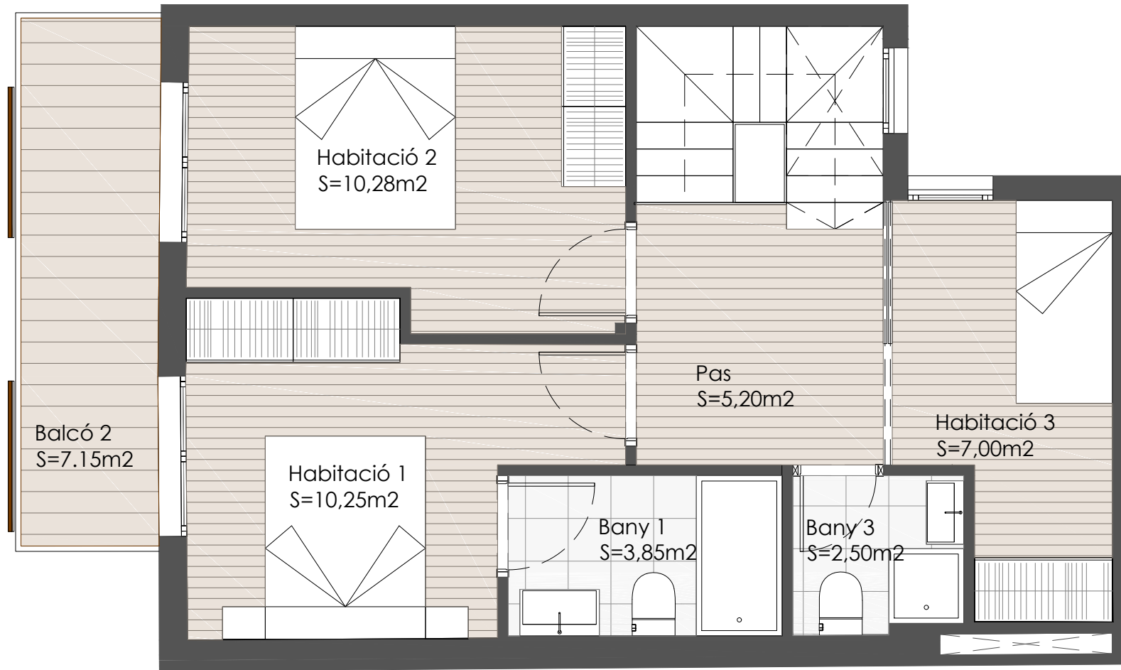
Planta Cinquena
