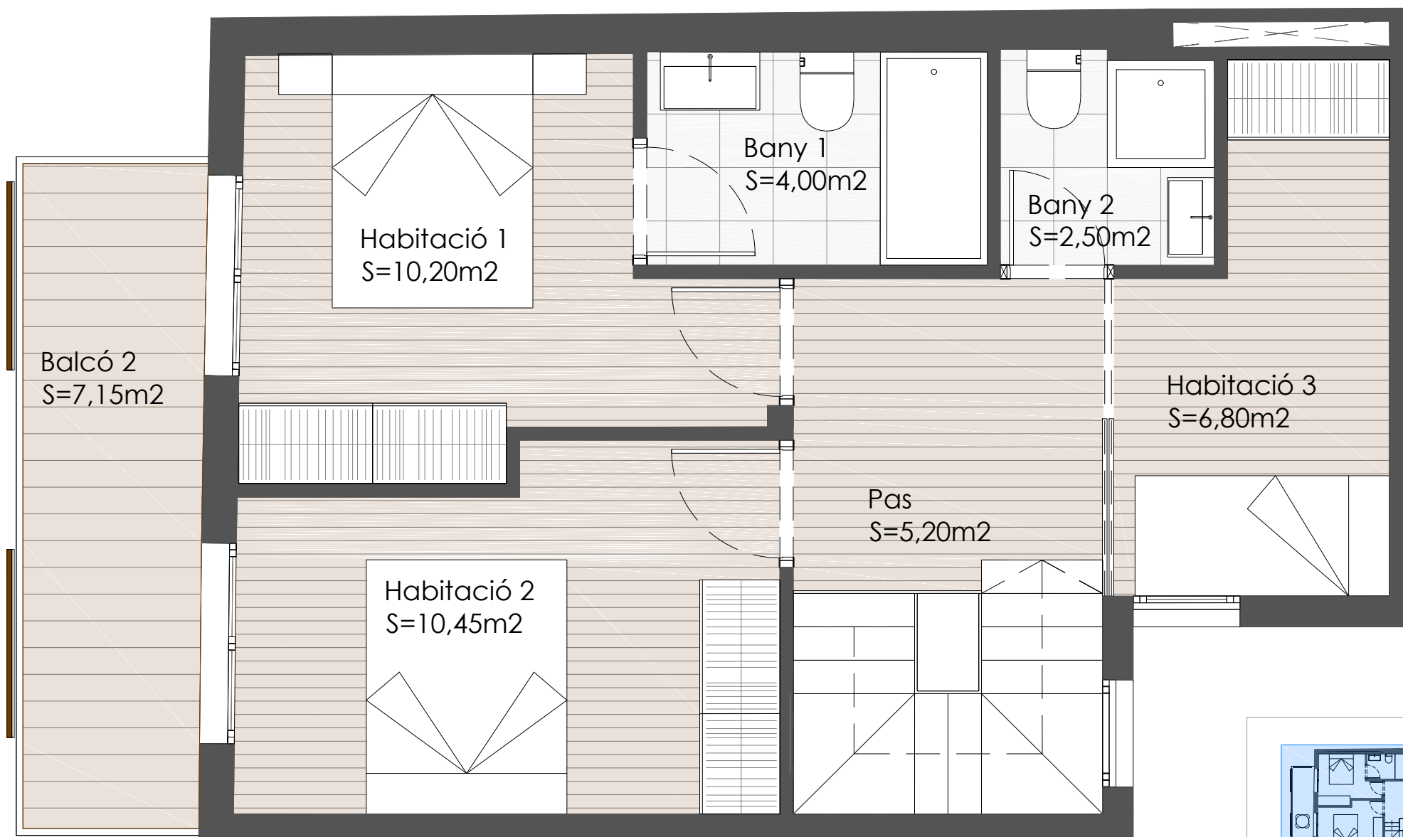
Planta Cinquena
